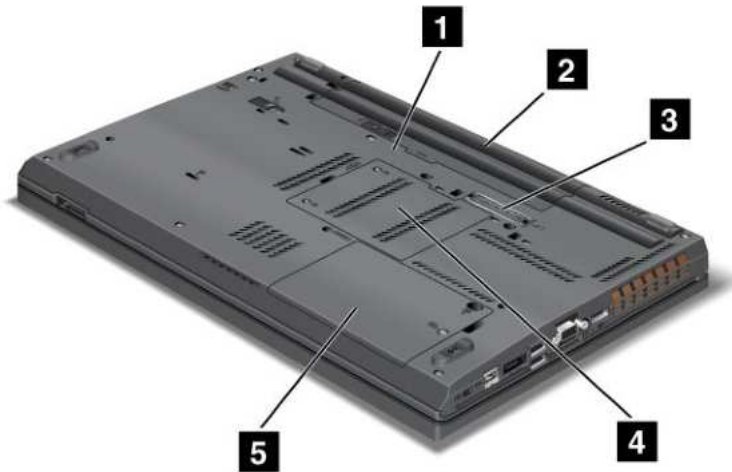
Abbildung 4. Abbildung: Ansicht des ThinkPads T520, T520i und W520 von unten
